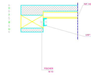
presjek B-B M 1:25
