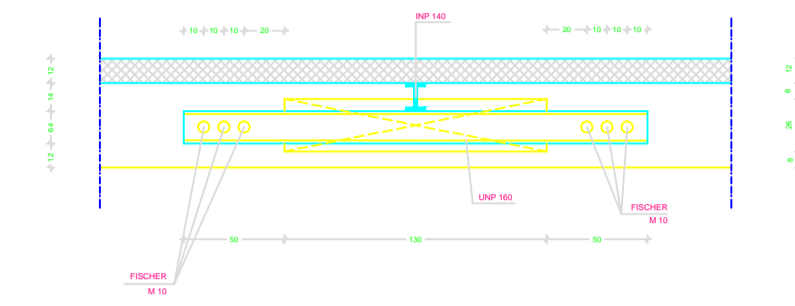
presjek C-C M 1:25
